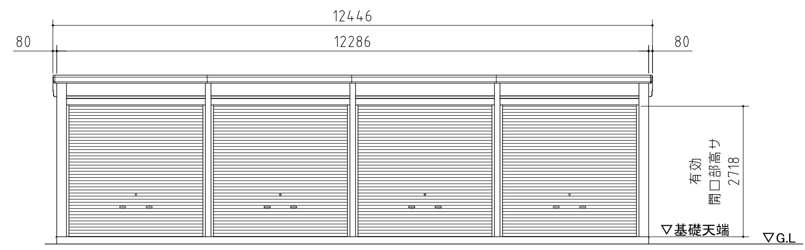
正面図
